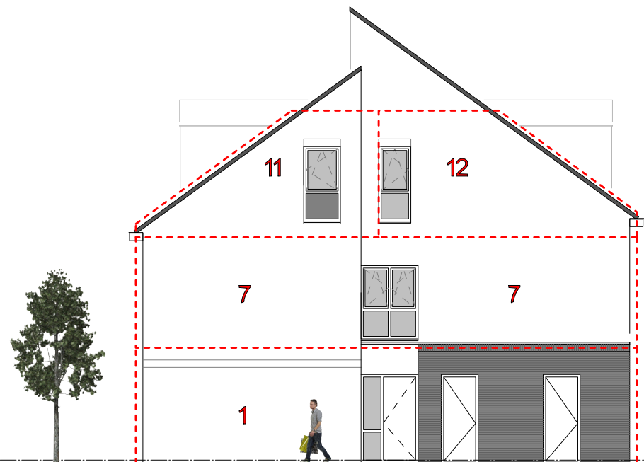
-Zijgevel Europalaan-
